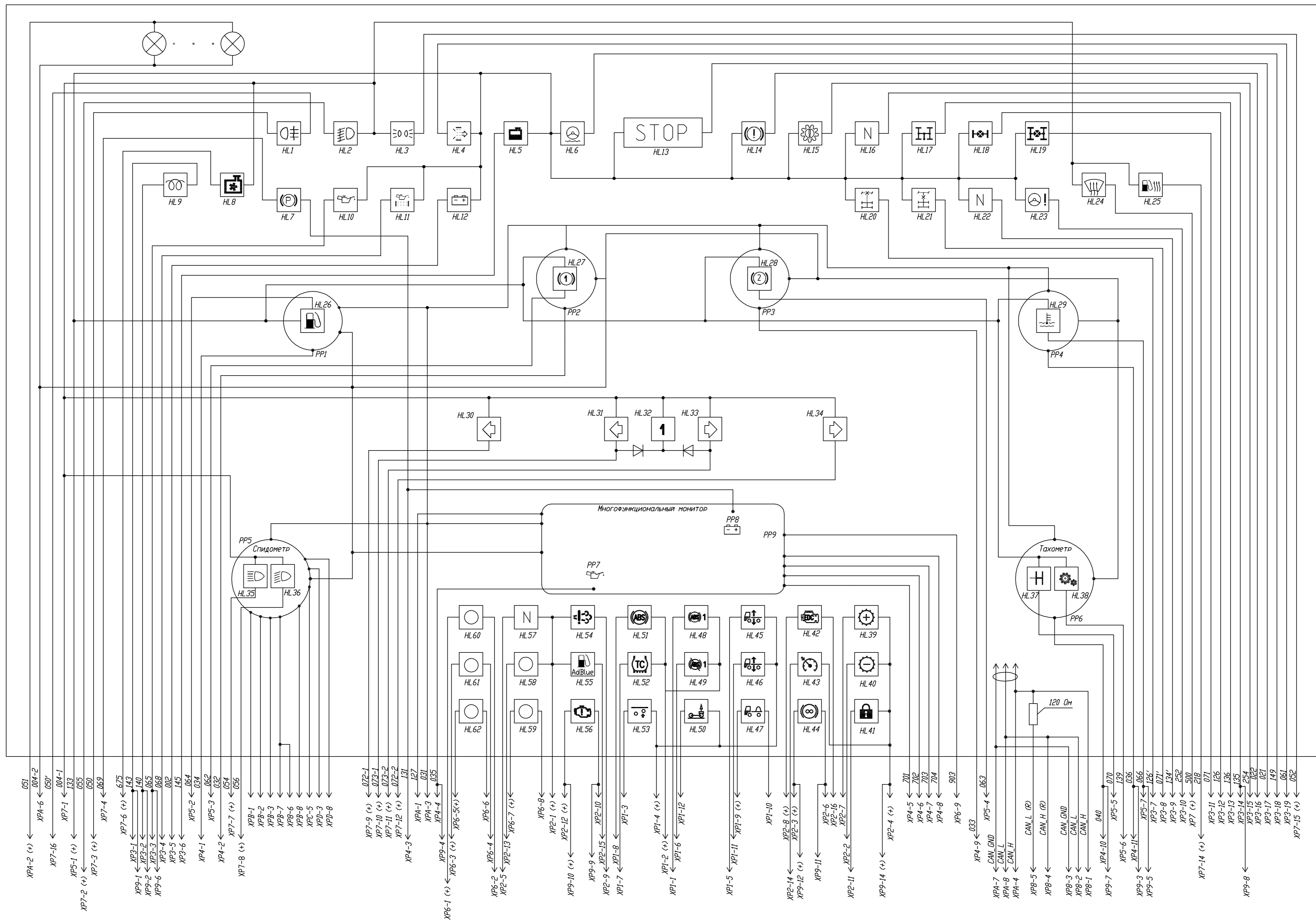
Рис.3. Схема электрическая функциональная комбинации приборов
